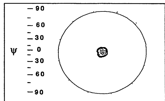
(b) (111) poles
