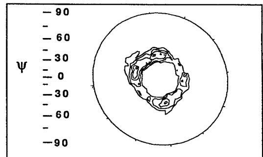
(b) (111) poles
